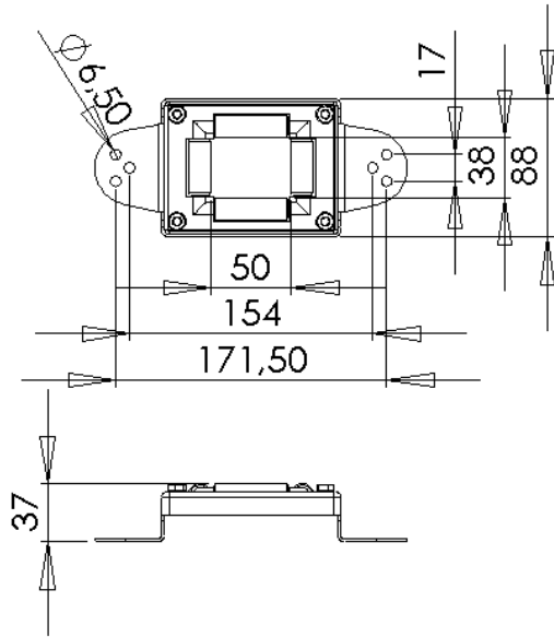
Wandblende Type WB1
