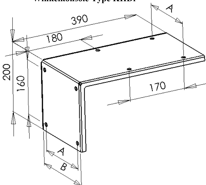
Winkelkonsole Type KHDr
