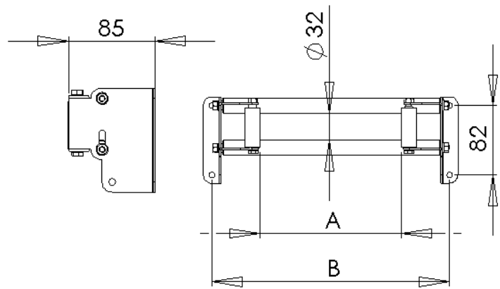
Schlaucheinlauffenster Type EFW2 + EFW3
